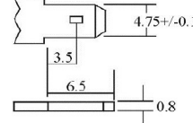
Optional Terminal F1 (Fasten Tab No.187E)
